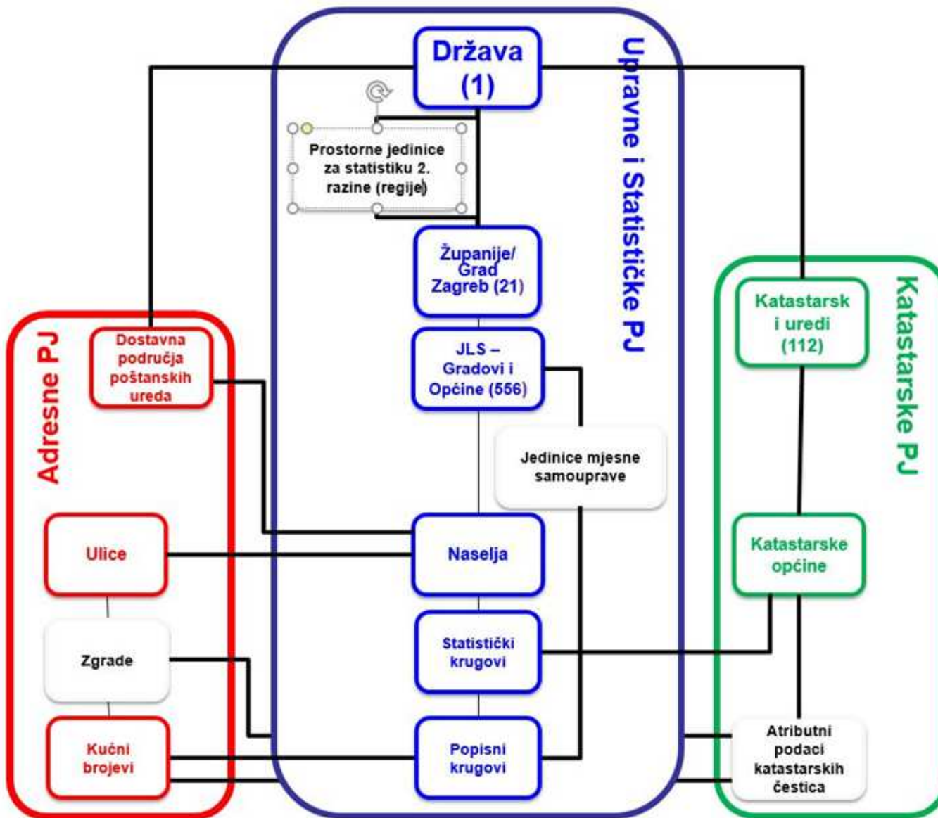
Model podataka registra prostornih jedinica
