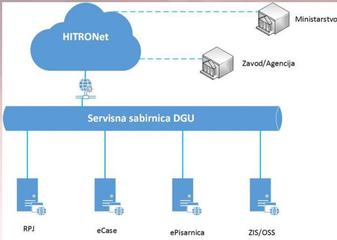
Servisna sabirnica DGU
